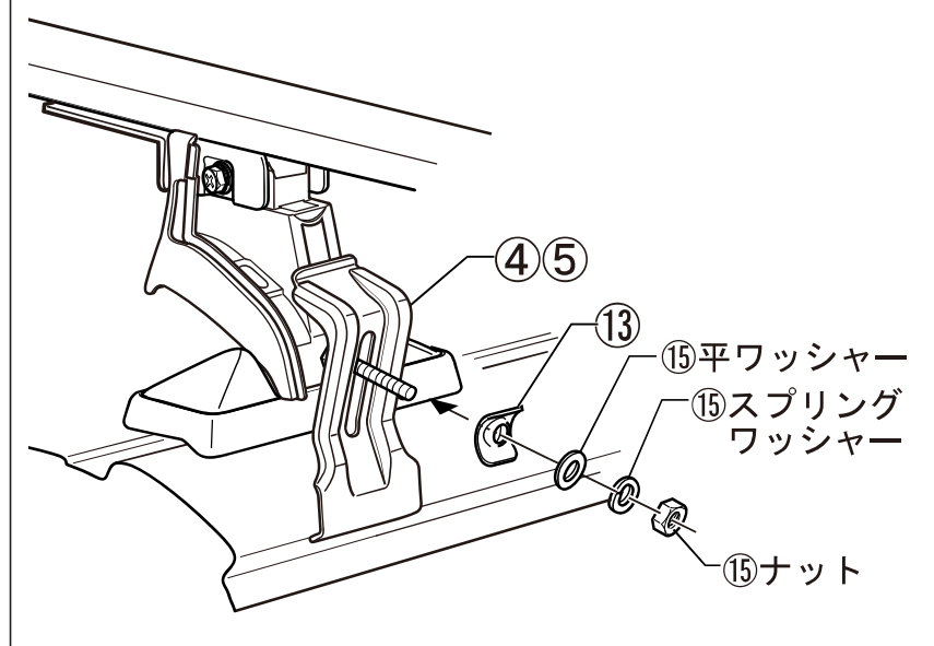
側面図
