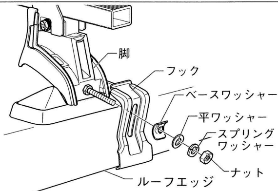
側面図 ルーフモール有車の場合
